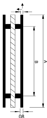
Retangular Plano 25x08x400 mm Escovado ref.: 377
